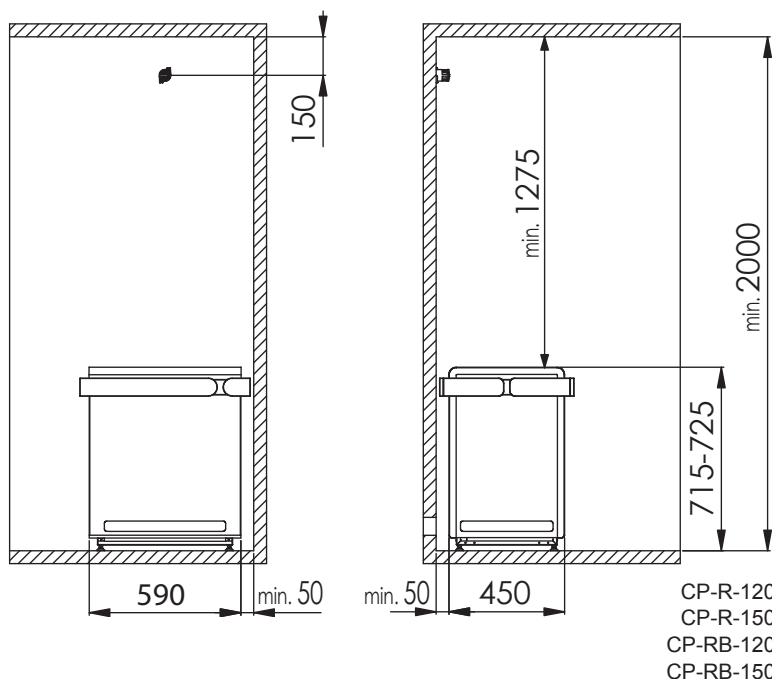
afb. 2 Veiligheidsafstanden Concept R 12 kW en 15 kW (CP-R-120 / CP-R-150 / CP-RB-120 / CP-RB-150) maten in mm
