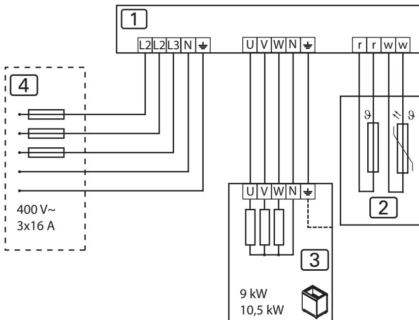
Bild 3 Kopplingsschema Concept R 9 kW och 10,5 kW (CP-R-090 / CP-R-105 / CP-RB-090 / CP-RB-105)
