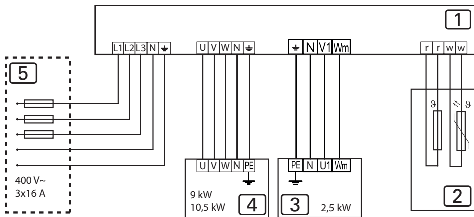
Bild 2 Elschema Concept R Combi 9 kW och 10,5 kW
