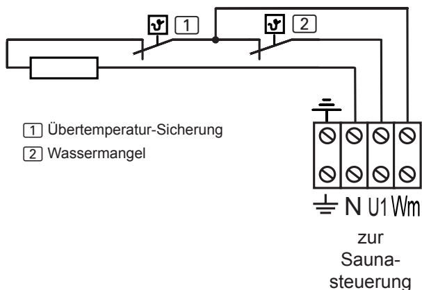
Abb.4 Verdrahtungsschema - Verdampfer
