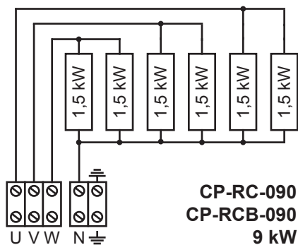
SI. 3 Sheme priključitve in ožičenja - ogrevalni sistem
