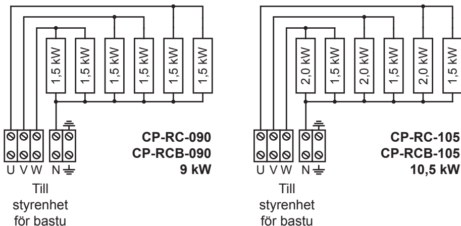
Bild 3 Kopplingsscheman – värmesystem
