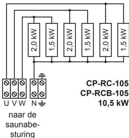
Afb. 3 Bedradingsschema's – Verwarmingssysteem
