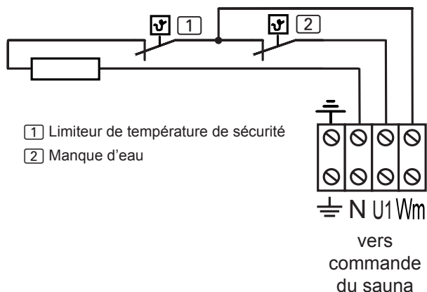
Fig. 4 Schéma de câblage – évaporateur
