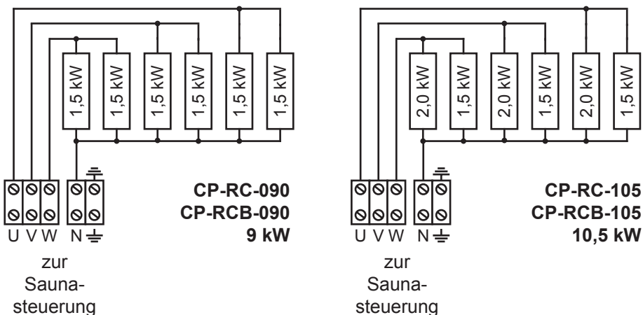
Abb.3 Verdrahtungsschemen - Heizsystem
