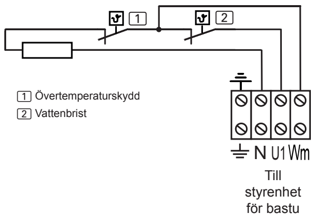
Bild 4 Kopplingsschema – förångare
